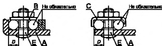
Рисунок 2б — Шпильчные зажимы
