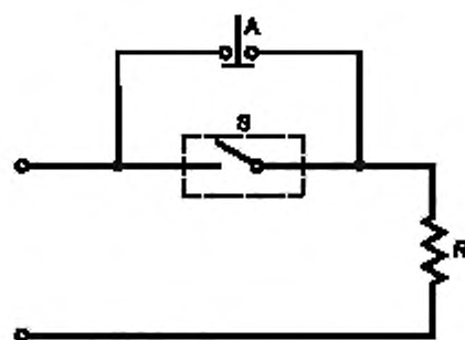
A — вспомогательный выключатель для установления нагрузки выключателя; R — активная нагрузка; S — испытуемый образец
