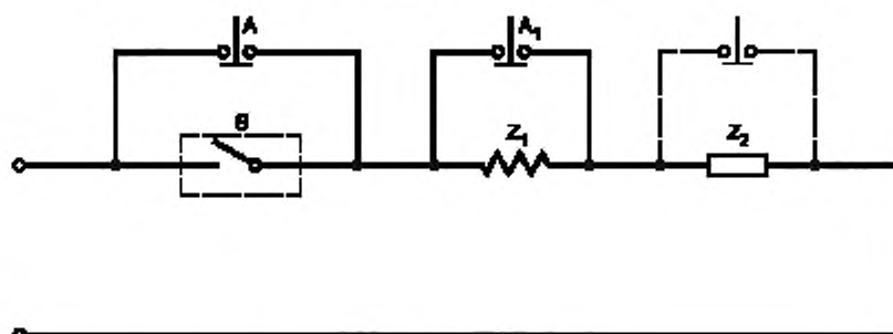
A — вспомогательный выключатель для установления нагрузки выключателя; A 1 — вспомогательный выключатель для получения тока «размыкания»; S — испытуемый образец; Z 1 — активная нагрузка для тока размыкания; Z 2 — нагрузка для тока замыкания.
