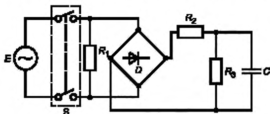
Рисунок 8 — Испытательное гнездо плоского вторичного соединителя
