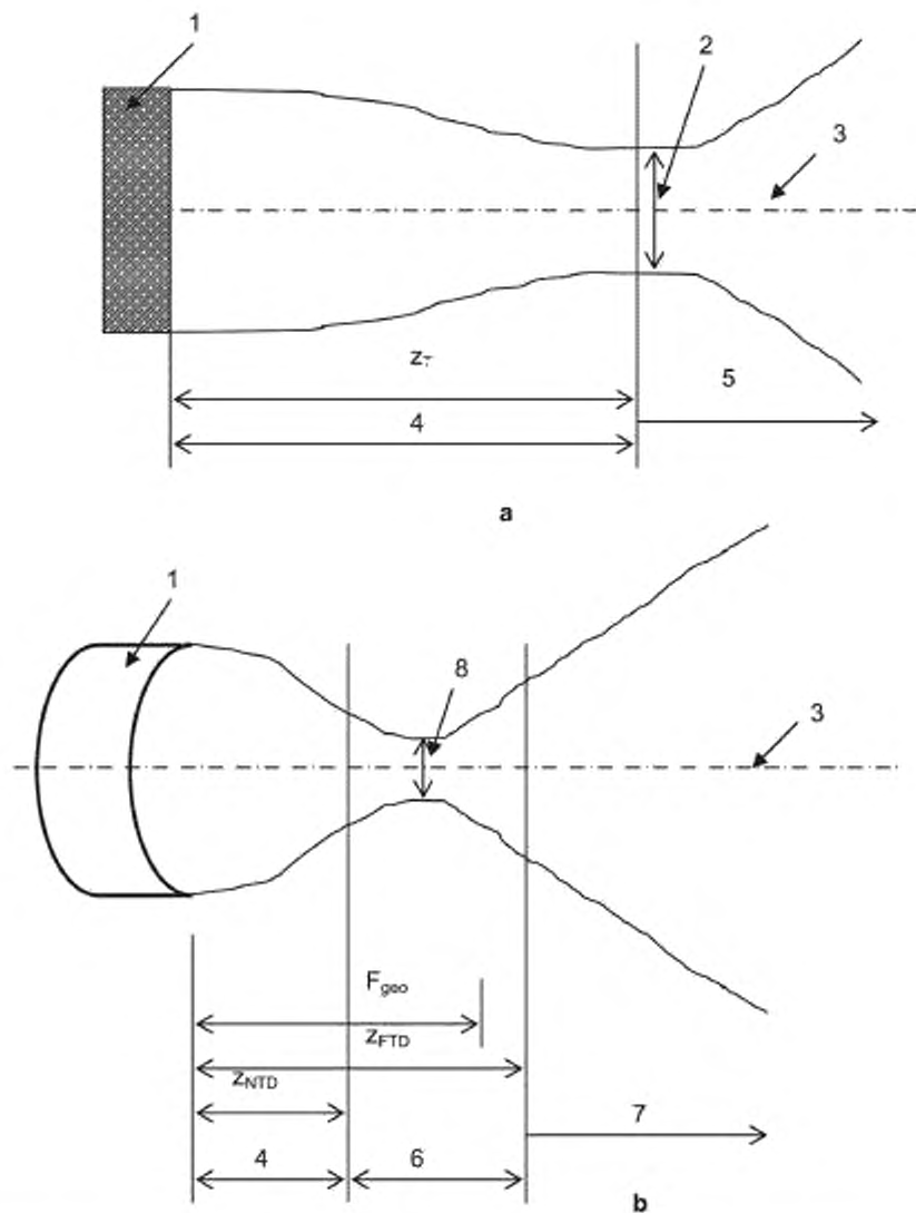
1 — преобразователь; 2 — минимальная ширина пучка (на уровне минус 6 дБ) в естественном фокусе; 3 — ось пучка; 4 — зона Френеля (ближнее поле); 5 — зона Фраунгофера (дальнее поле); 6 — фокальная зона Фраунгофера; 7 — зона Френеля (дальнее поле); 8 — минимальная ширина пучка (на уровне минус 6 дБ) в созданном фокусе; z_T — переходный интервал; F_{geo} — геометрическое фокусное расстояние; z_{NTD} — ближний переходный интервал; z_{FTD} — дальний переходный интервал
