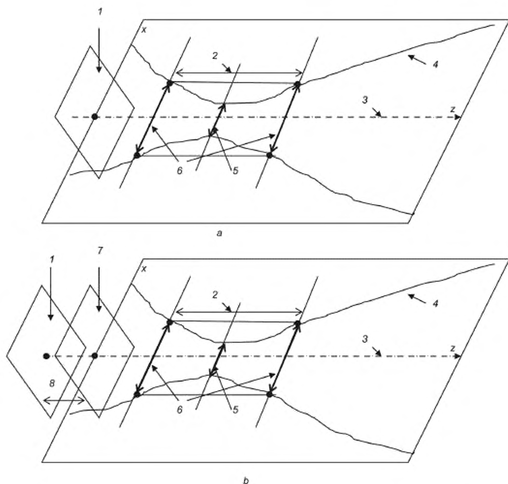
1 — внешняя апертура преобразователя; 2 — протяженность фокальной области; 3 — ось пучка; 4 — профиль пучка на уровне минус 6 дБ; 5 — минимальная ширина пучка W_{min} на уровне минус 6 дБ; 6 — ширина пучка, равная 2 W_{min} ; 7 — апертура источника; 8 — компенсированное расстояние
