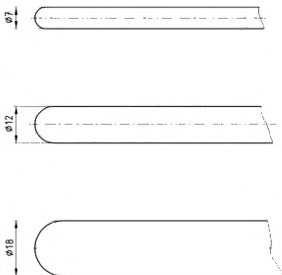
Рисунок 1 — испытательный палец
