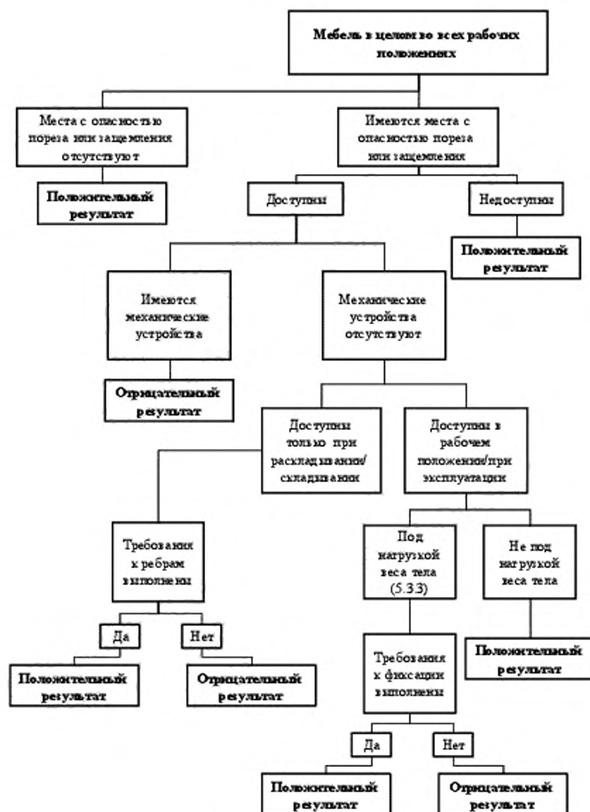
Рисунок А.1 – Схематическое представление требований к местам, представляющим опасность пореза или защемления
