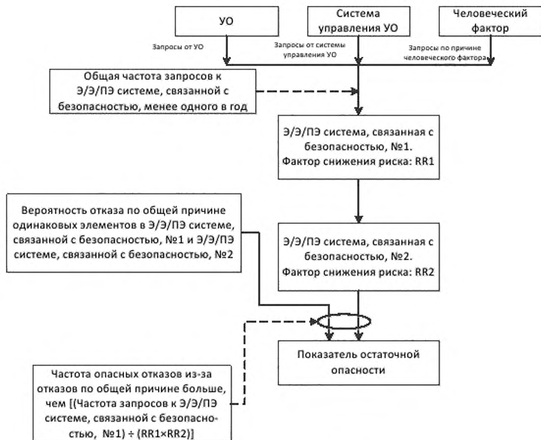
Рисунок А.6 – Общая причина между двумя Э/Э/ПЭ системами, связанными с безопасностью
