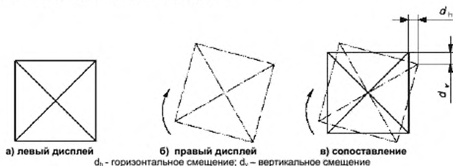
Рисунок Е.4 - Межглазная разность вращения
