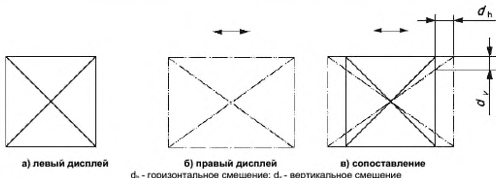
Рисунок Е.7 – Межглазная разница горизонтального увеличения
