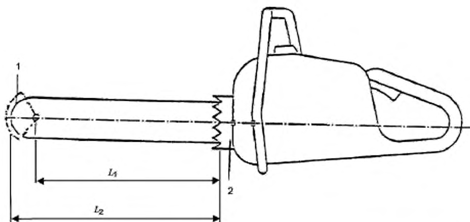
Рисунок 101 — Терминология цепных пил
