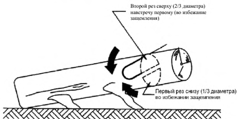
Рисунок ВВ.105 — Хлыст опирается одним концом
