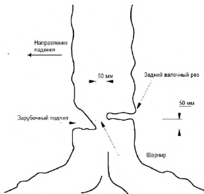
Рисунок ВВ.102 — Описание валки: подпиливание
