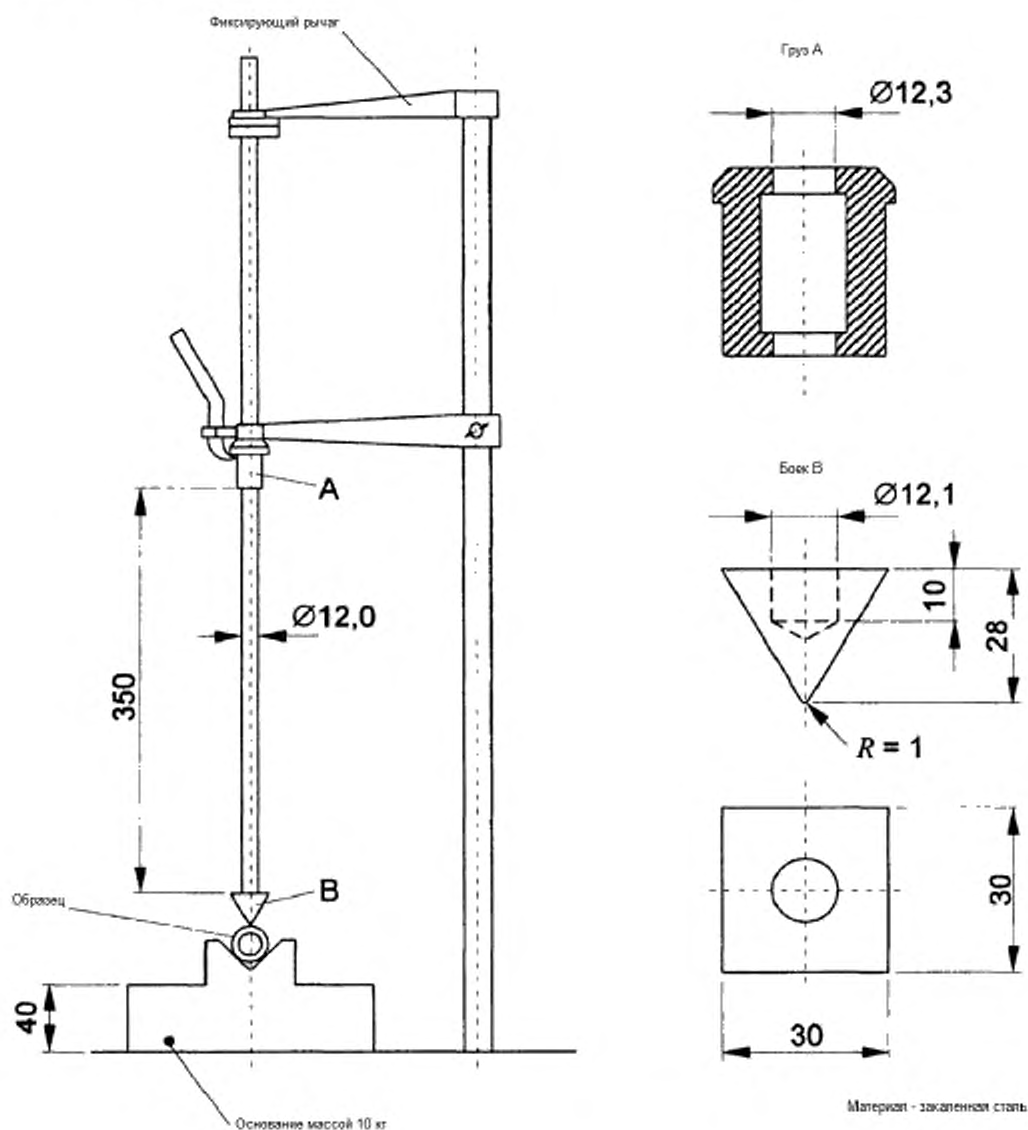
Рисунок 110 — Стенд для ударных испытаний изоляции рукоятки
