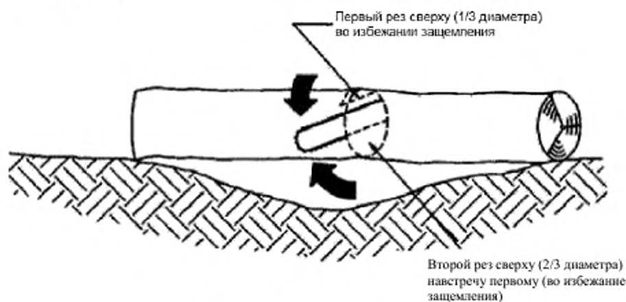
Рисунок ВВ.106 — Хлыст опирается обоими концами
