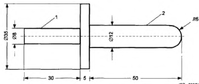
1 — рукоятка; 2 — рабочая часть
