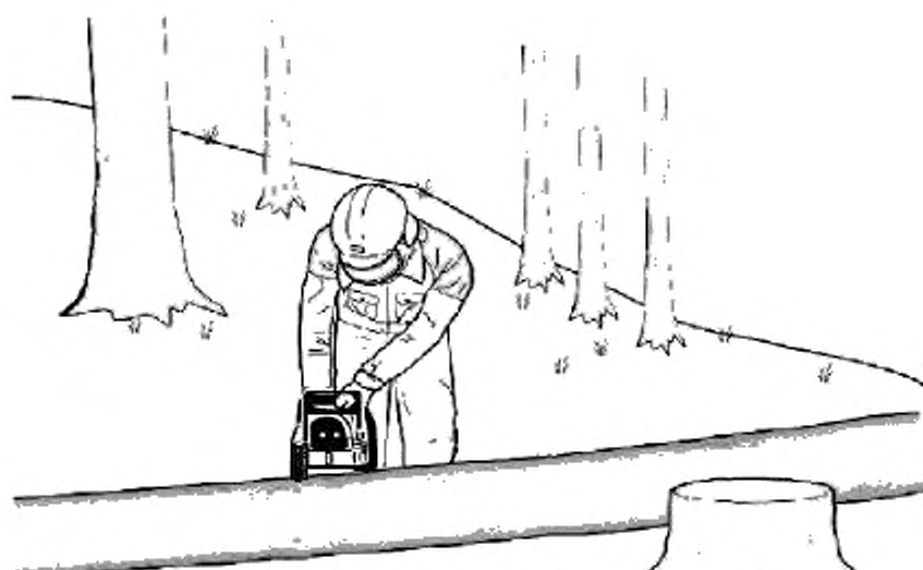
При резке стоять на верхней стороне, так как хлыст может покатиться
