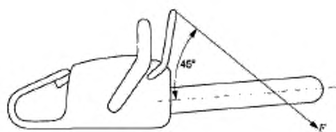
Рисунок 107 — Статическое испытание усилия спуска тормоза
