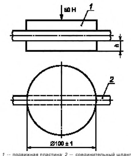
Рисунок 1 — Схема испытания
