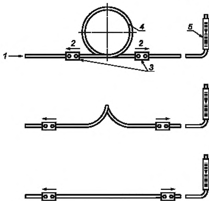
1 — подача воздуха; 2 — направление движения; 3 — зажимы; 4 — шланг; 5 — ротаметр
