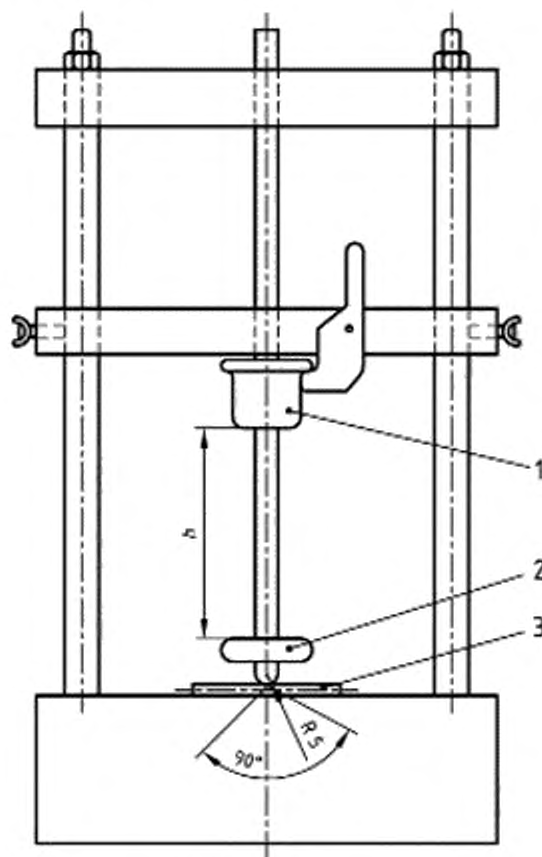
1 – молот, 2 – прокладка из закаленной стали, 3 – образец
