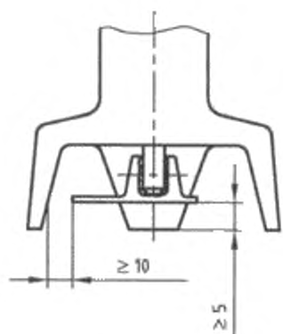
Рисунок 5 – Неподвижное защитное ограждение со стороны привода
