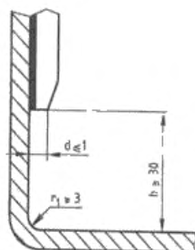
Рисунок В.9 – Пищевая зона
