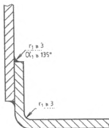
Рисунок В.8 – Пищевая зона
