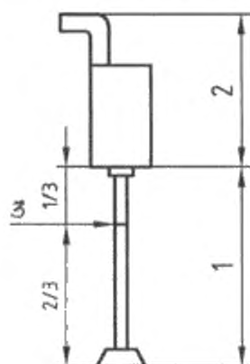
1 – пищевая зона; 2 – непищевая зона; 3 – метка, указывающая на глубину погружения рабочего органа
