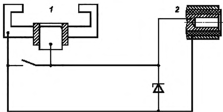
1 — колодка; 2 — гнездо (розетка)
