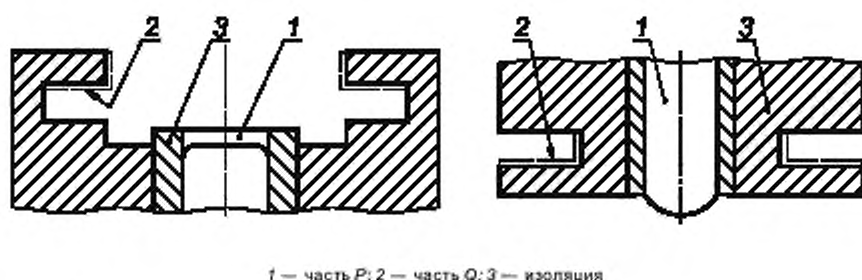
1 — часть P ; 2 — часть Q ; 3 — изоляция
