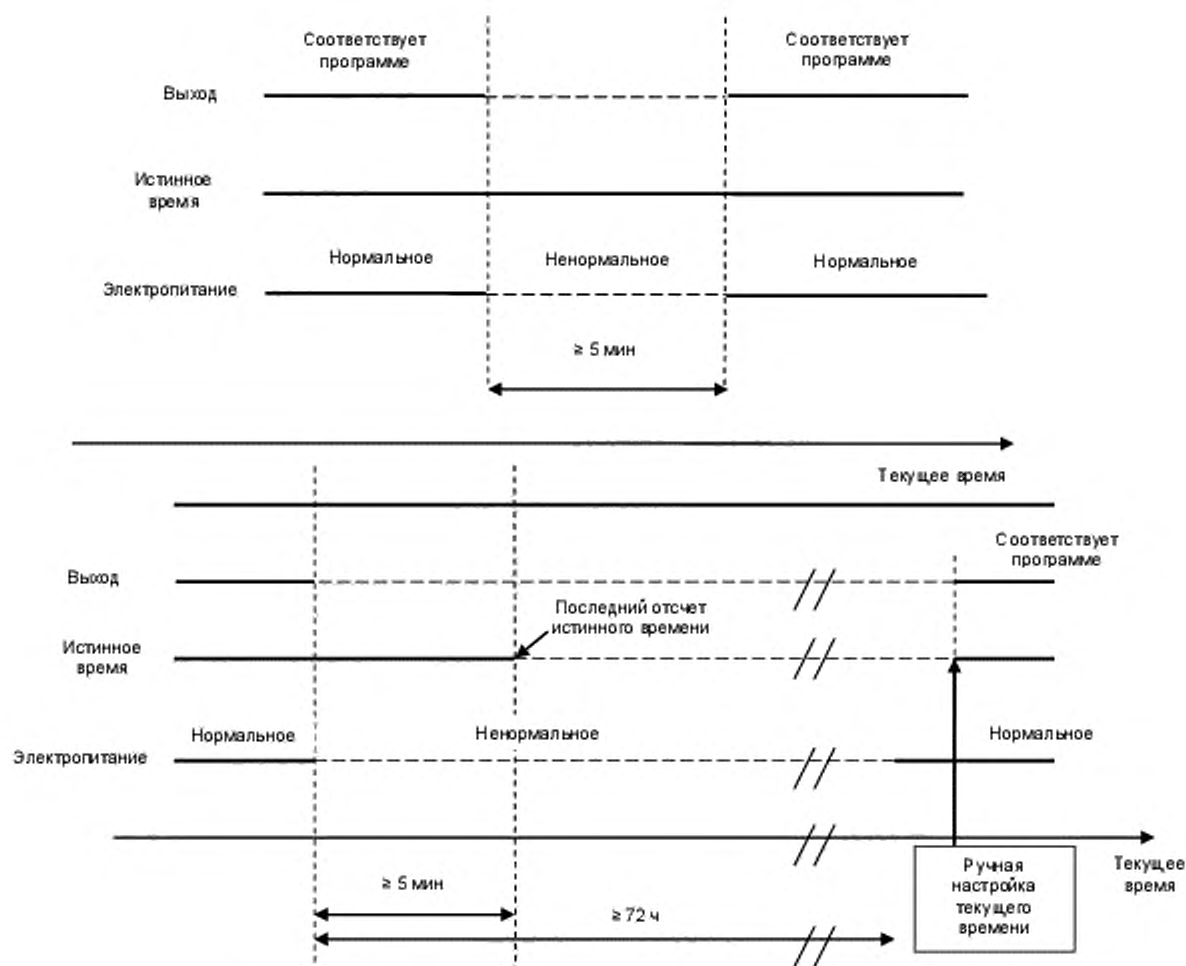
Рисунок 7 – Временная диаграмма защиты данных
