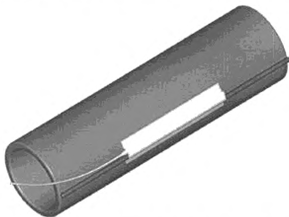
Рисунок 8 — Датчик ограничителя температуры на поверхности электронагревателя
