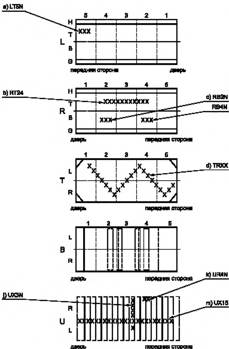
Рисунок С.1 — Примеры расположения кодов на контейнере, Лист 1
