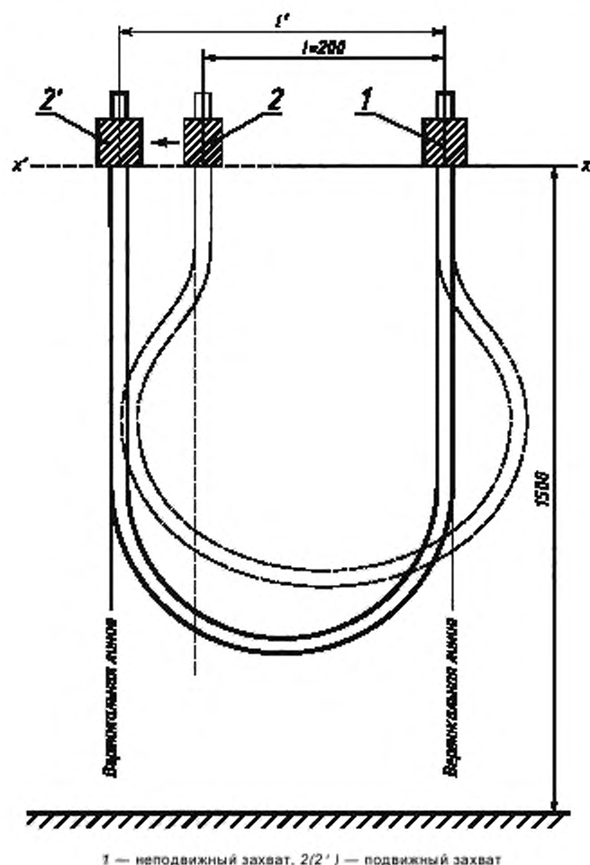
Рисунок 3 — Испытание на статическую гибкость
