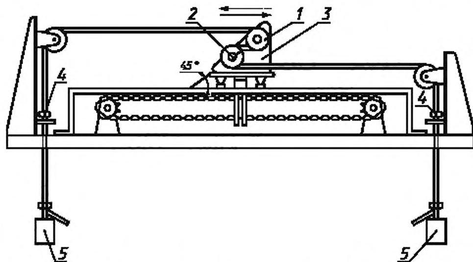
1, 2 — ролики; 3 — каретка; 4 — удерживающие зажимы; 5 — груз
