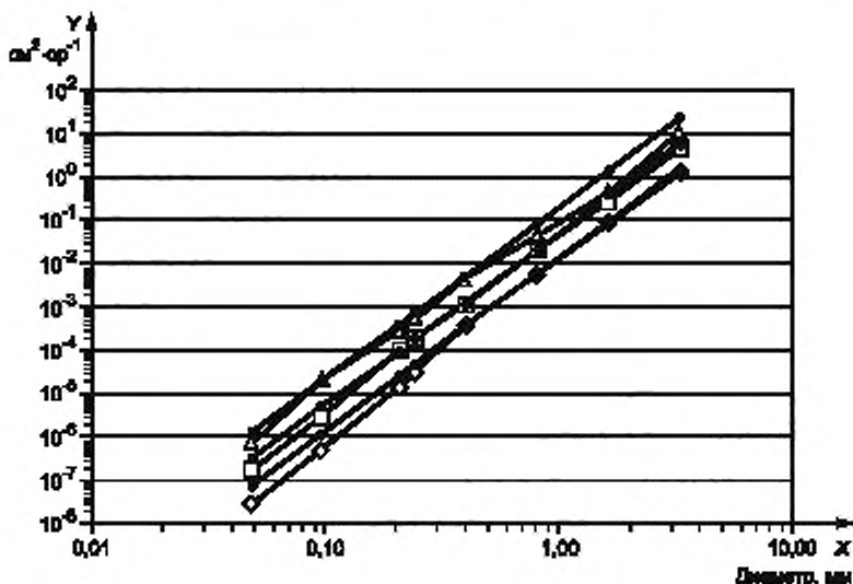
Рисунок В.4 — Зависимость экспериментально полученных значений площади поперечного сечения обратного рассеяния от плоского торца проволоочек из нержавеющей стали от их диаметра на частотах 9,6 МГц (Δ), 4,8 МГц (·) и 2,4 МГц (◇) [29]
