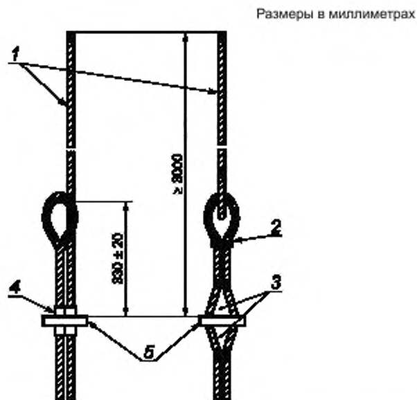
1 — вспомогательный удлинительный канат; 2 — бензель (типовая); 3 — клин; 4 — механическое зажимное приспособление; 5 — балясина
