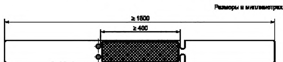
Рисунок 4 — Удлиненная балясина люцманского штурмтрапа
