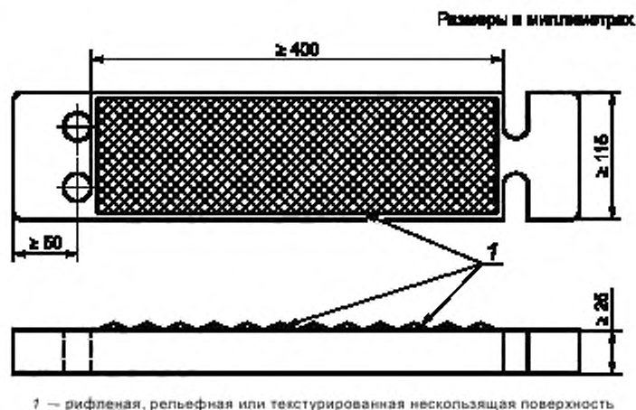
Рисунок 2 — Типичная балясина штормтрапа с указанием возможных вариантов отверстий и вырезов
