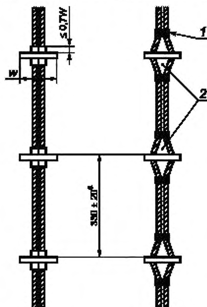
1 — бензель (типовой), 2 — клинья. a — стандартное значение
