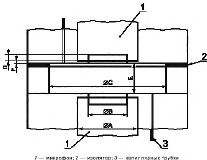
Рисунок С.2 — Эскиз камеры большого объема
