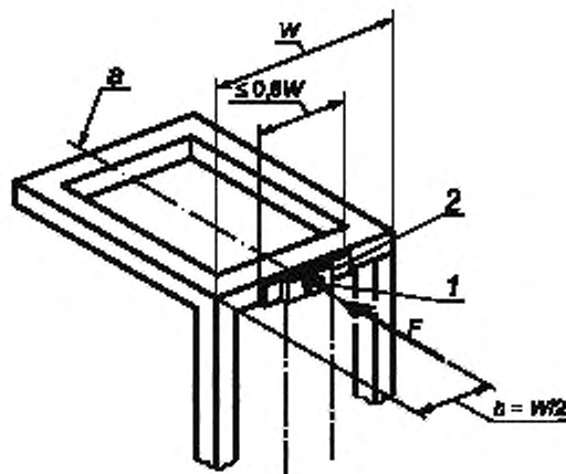
1 — упор со сферическим углублением; 2 — распределитель нагрузки; \alpha — ось, параллельная продольной оси машины
