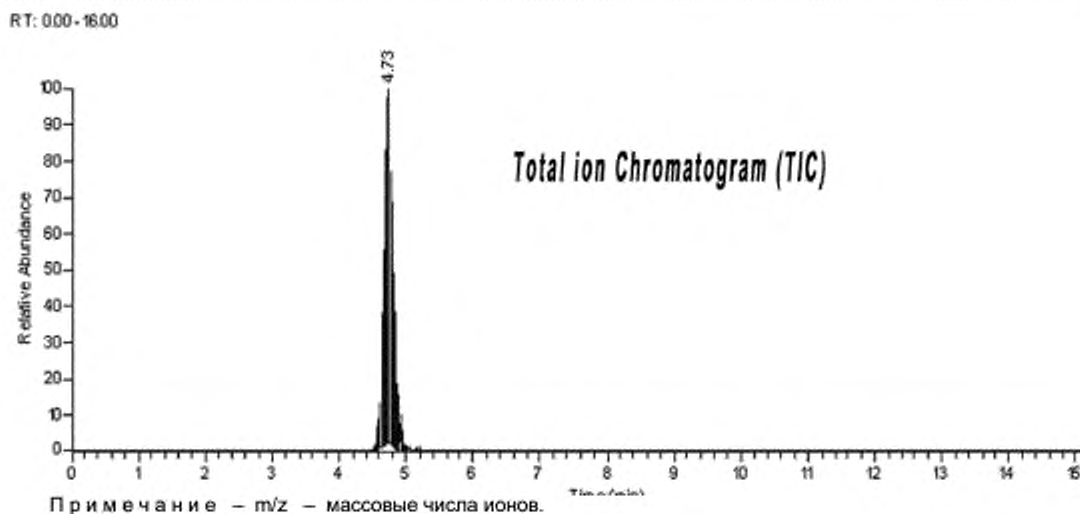
Рисунок В.2 — Хромограмма LC-MS/MS циануровой кислоты (CA) из экстракта детской молочной смеси NIST при концентрации введенного вещества: CA = 0,50 мг/кг
