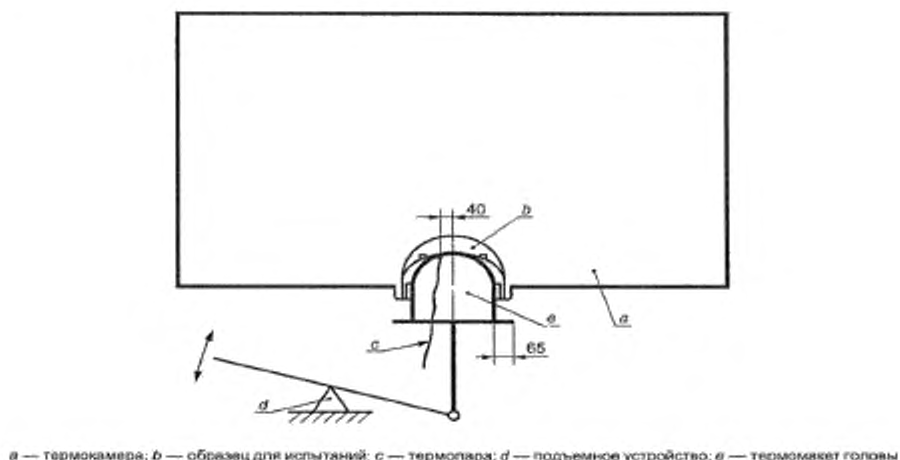
Рисунок 2 — Упрощенное изображение термокамеры
