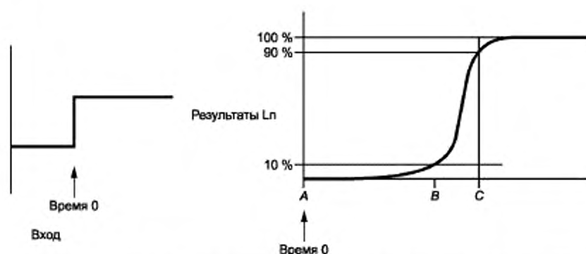
Рисунок 1 – Время срабатывания (чувствительность всей системы)
