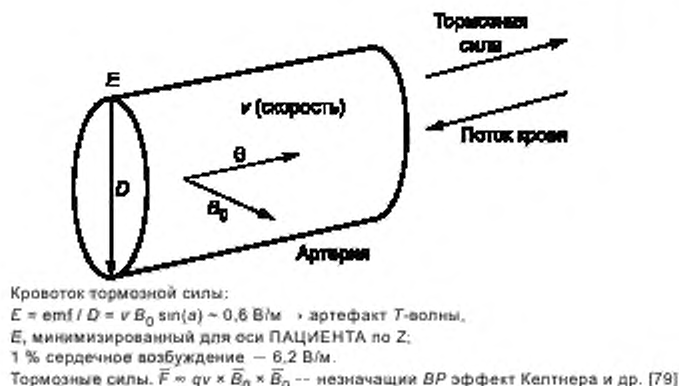
Рисунок ВВ.1 — Постоянное магнитное поле: потенциалы потока
