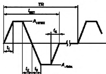
t_1 , t_2 , t_3 , t_4 — длительности фронта и среза биполярных импульсов; t_{кл} — время включения; TR — период процесса; A_{+max} и A_{-max} — максимальный градиент силы
