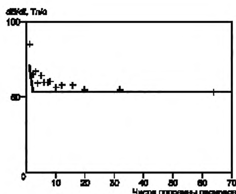
Рисунок ВВ.7 — Пороговые значения dB/dt для формы волны градиента синусоиды как функция числа половин периодов в форме волны
