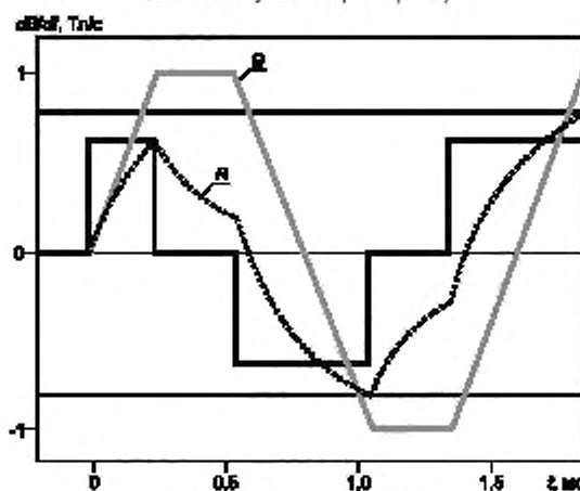
Рисунок BB.4 — Значение ответа R(t) , произведенного скручиванием прямоугольного стимула dB/dt , и функций ответа импульса нерва n(t - \theta)
