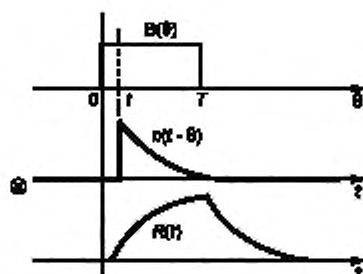
Рисунок BB.4 — Значение ответа R(t) , произведенного скручиванием прямоугольного стимула dB/dt , и функций ответа импульса нерва n(t - \theta)
