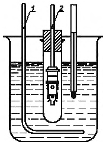
1 — мешалка; 2 — линия погружения
