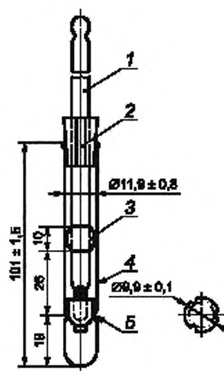
1 — термометр; 2 — прорезь в пробке для вентиляции; 3 — направляющая пробка для обеспечения необходимого зазора между термометром и пробкой; 4 — пробка из боросиликатного стекла; 5 — три равномерно расположенных углубления для удержания чашки
