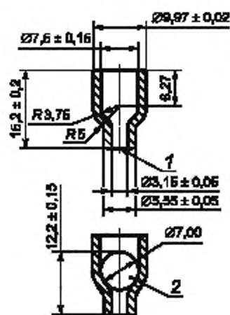
1 — острый край (удалены только заусенцы); 2 — стальной шарик
