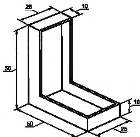
Рисунок А.7 — Бокс с двумя прямоугольными ящиками
