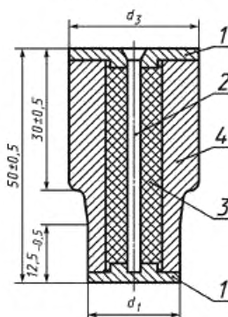
Типоразмеры DII, DIII
