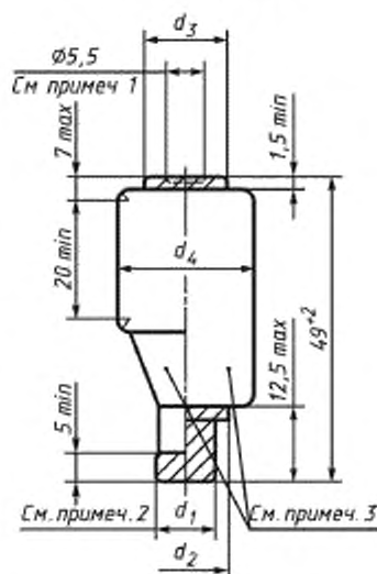
Типоразмеры DII; DIII
