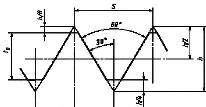
Метрическая резьба ИСО
