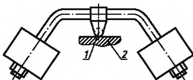
Рисунок 17 — Испытательное устройство для вдавливания шарика
