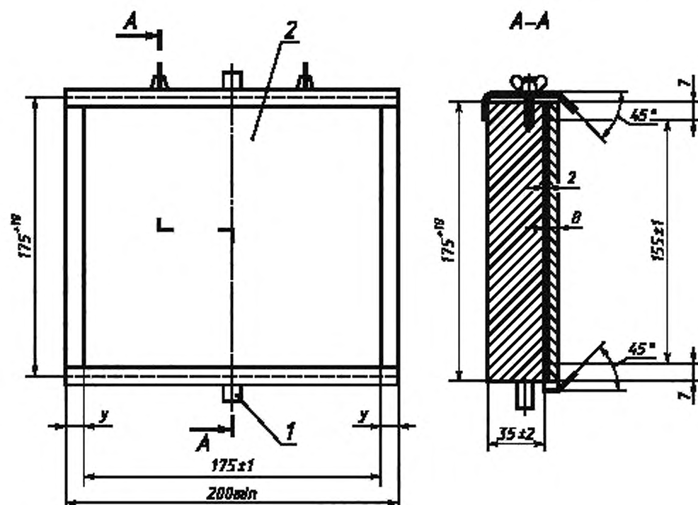
Рисунок 16 — Монтажная опора
