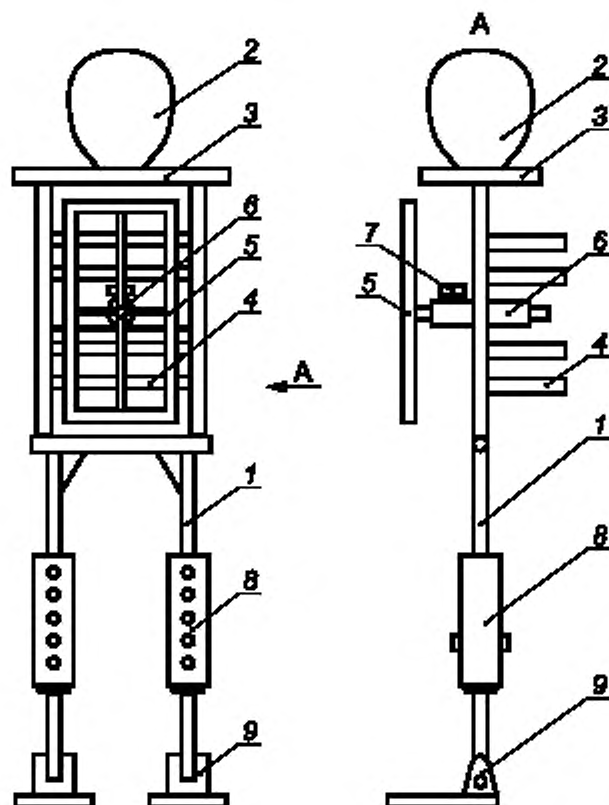
1 — осто́в мане́кена; 2 — муля́ж голо́вы че́ловека; 3 — плече́вой ка́ркас; 4 — габа́ритная ско́ба; 5 — габа́ритная ра́мка; 6 — на́правляющая вту́лка; 7 — сто́порный ви́нт; 8 — регуля́тор вы́соты мане́кена; 9 — подо́шва
