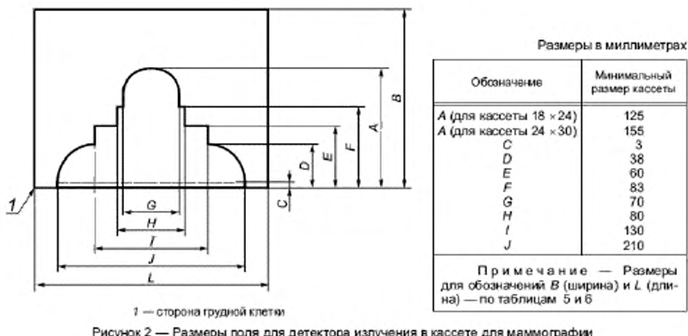
Рисунок 2 — Размеры поля для детектора излучения в кассете для маммографии
