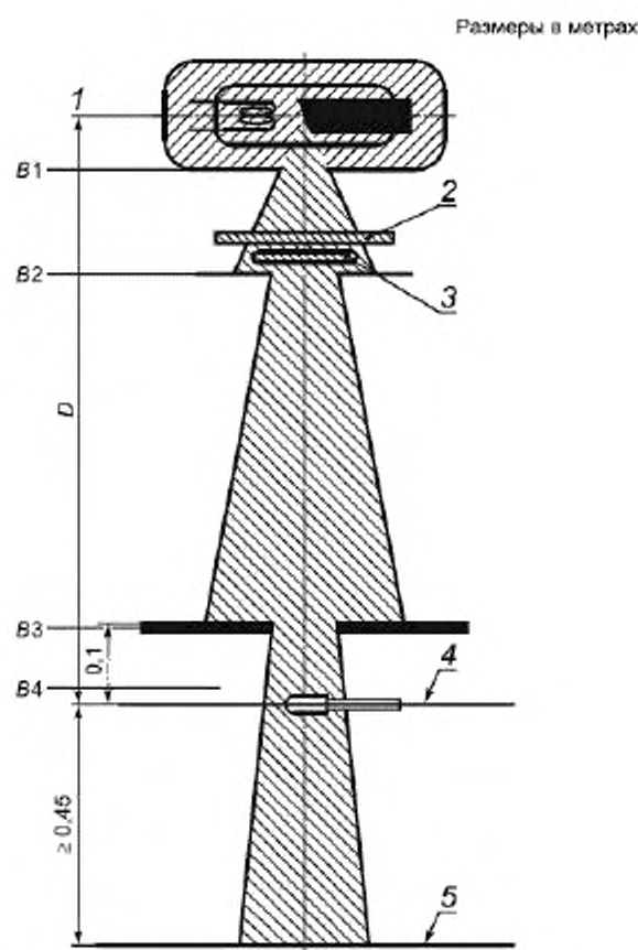
1 — диафрагмы пучка излучения (B1, B2, B3, B4), 2 — дополнительный фильтр, 3 — контрольный детектор (R1); 4 — измерительный детектор (R2); 5 — щит из свинца; D — переменное расстояние
