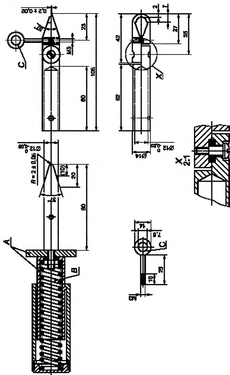
A — изоляционный материал; В — диаметр пружины; С — петля
