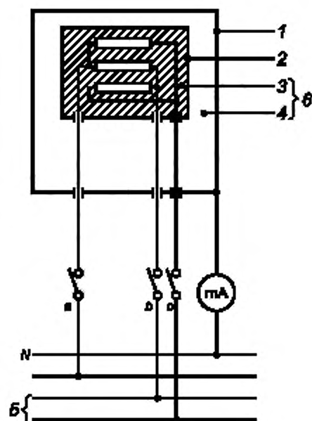
1 — доступная часть; 2 — недоступная металлическая часть; 3 — основная изоляция; 4 — дополнительная изоляция; 5 — трехфазное питание; б — двойная изоляция
