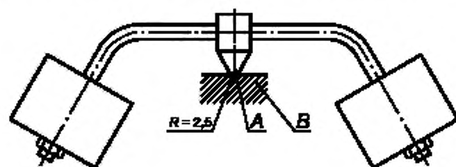
А — сферическая часть; В — испытуемый образец
