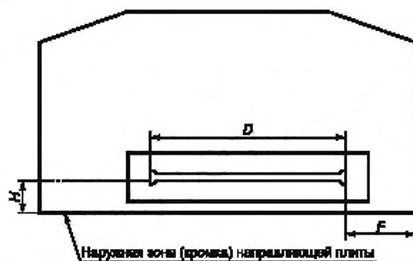
Рисунок 113 — Основные размеры направляющей плиты
