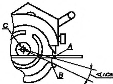
А — точка пересечения окружности вершин зубьев пильного диска с нижней поверхностью направляющей плиты; В — точка пересечения окружности вершин зубьев пильного диска с ортогональной проекцией на плоскость диска от каждой стороны или от передней кромки подвижного защитного кожуха в зависимости от того, что дает большее значение угла ACB; С — центр пильного диска
