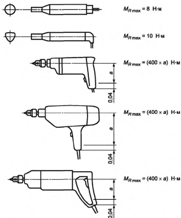
Рисунок 102 — Реактивный момент машин, удерживаемых одной рукой
