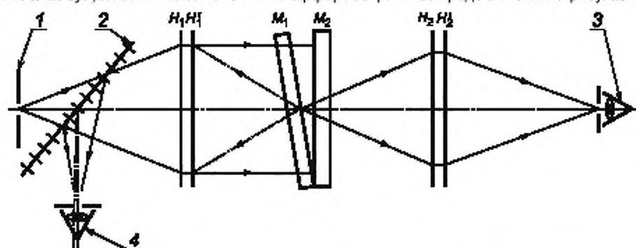
1 — излучатель; 2 — светоделитель; 3 — наблюдение прошедшего излучения; 4 — наблюдение отраженного излучения; H 1 H 1 , M 1 , M 2 , H 2 H 2 — плоские поверхности
