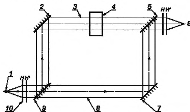
1 — излучатель; 2 — плоское зеркало; 3 — объектный пучок; 4 — испытываемый образец; 5 — светоделитель; 6 — наблюдатель; 7 — плоское зеркало; 8 — опорный пучок; 9 — светоделитель; 10 — коллиматор
