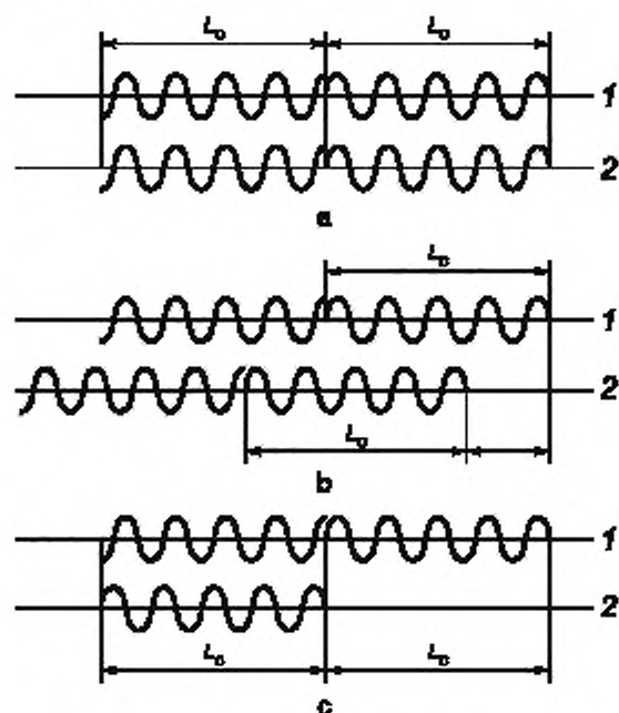
1, 2 — парциальные волны
