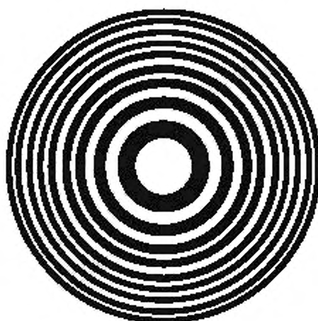
Рисунок 13 — Кольца Ньютона
