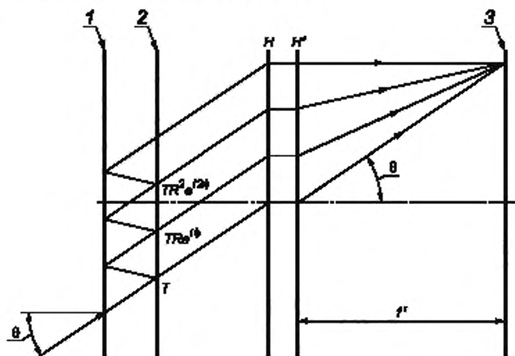
t — зеркало; 2 — зеркало; 3 — фокальная плоскость; HH' — линза
