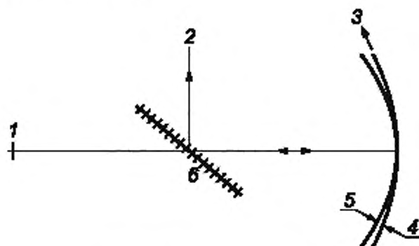
1 — излучатель; 2 — наблюдатель; 3 — воздушный зазор; 4 — испытываемая поверхность V ; 5 — пробная поверхность M (пробное стекло); 6 — светоделитель
