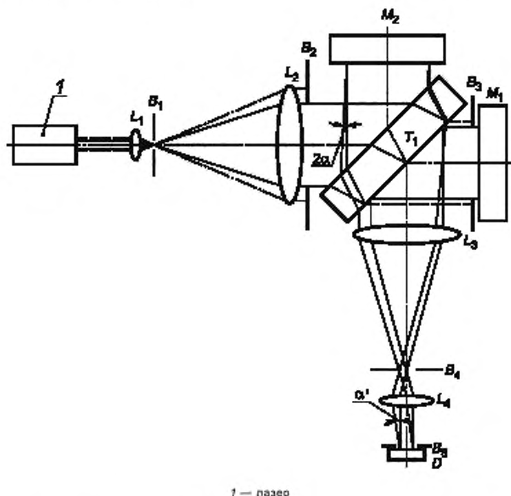
1 — лазер
