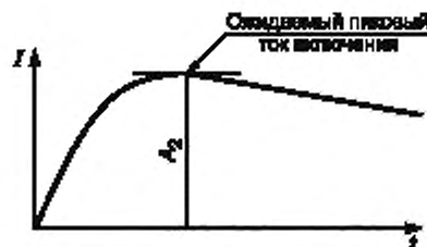
Рисунок 7b — Калибровка испытательной цепи для постоянного тока
