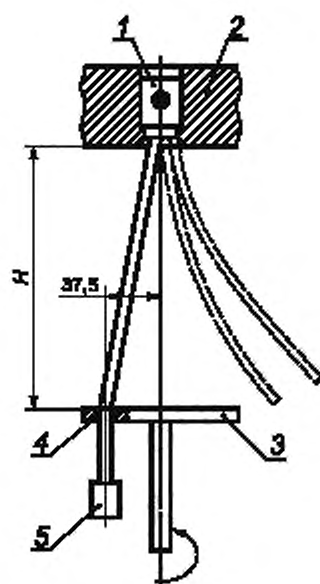
Рисунок 106 — Пример приложения усилия натяжения по оси зажима
