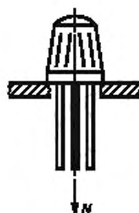
Рисунок 106 — Пример приложения усилия натяжения по оси зажима
