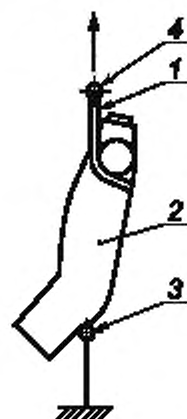
1 — спасательная петля; 2 — манекен корпуса; 3 — нижнее кольцо манекена корпуса; 4 — элемент крепления
