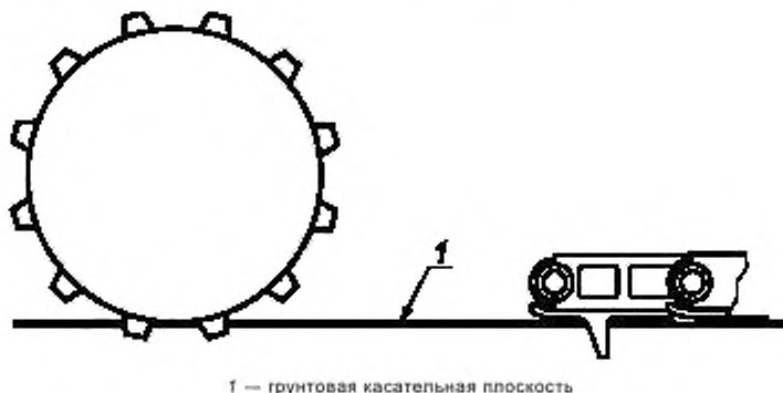
Рисунок 1 — Расположение грунтозацепов на поверхности грунта
