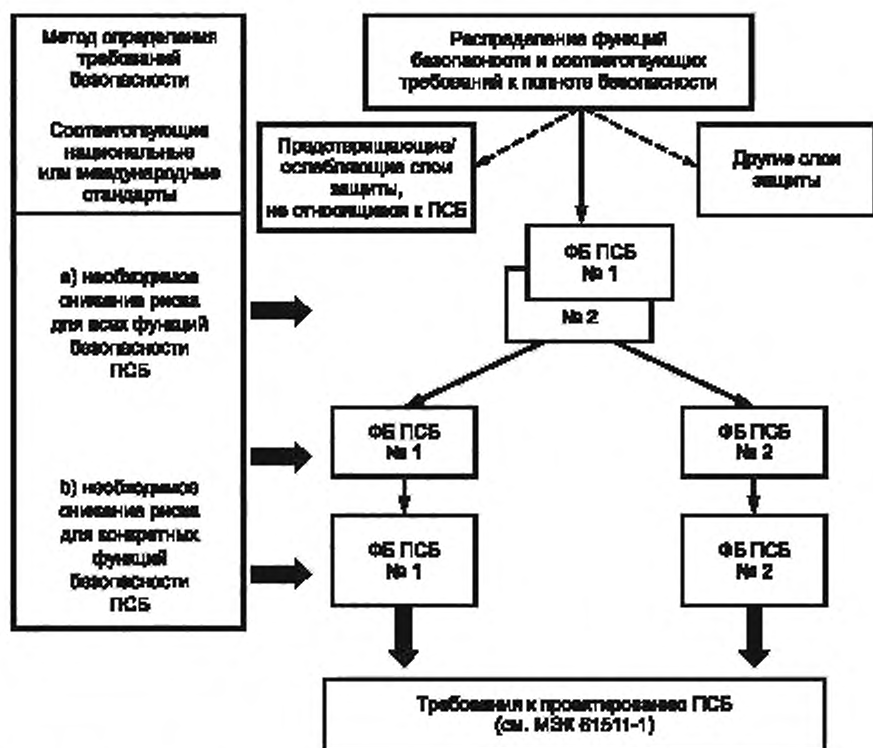
Рисунок 5 — Размещение требований безопасности по ПСБ, по слоям защиты или ослабления, не относящимся к ПСБ, и по другим слоям защиты
