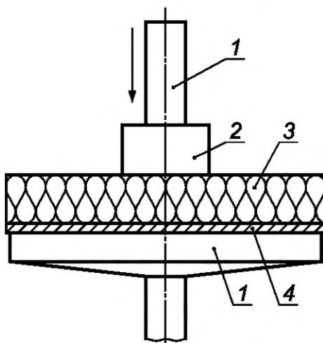
Рисунок 1 — Устройство для испытания
