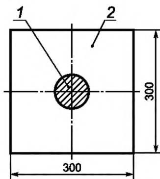
Рисунок 2 — Образец для испытания
