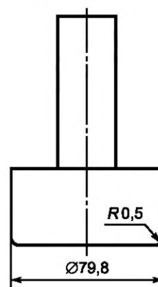
Рисунок 3 — Цилиндрический индентор
