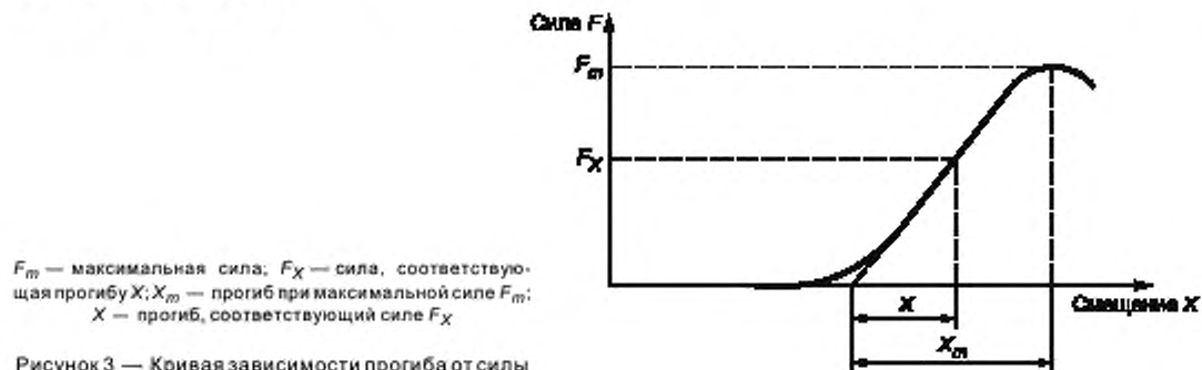
Рисунок 3 — Кривая зависимости прогиба от силы
