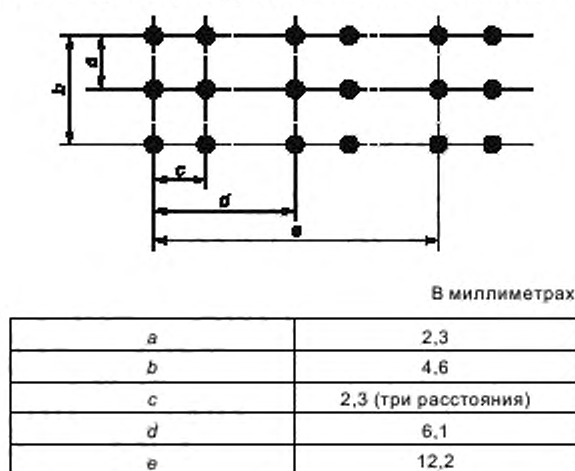
Рисунок 2 — Расположение точек ТИ
