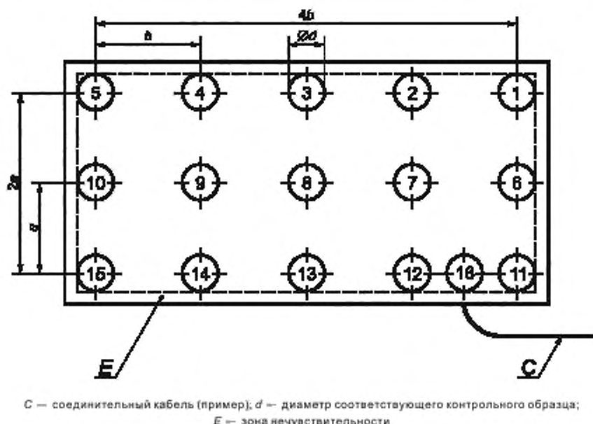
Рисунок 3 — Места испытаний эффективной чувствительности области одиночного датчика
