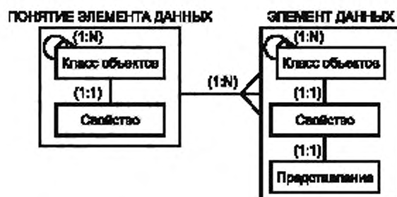
Рисунок 1 — Базовая модель элементов данных
