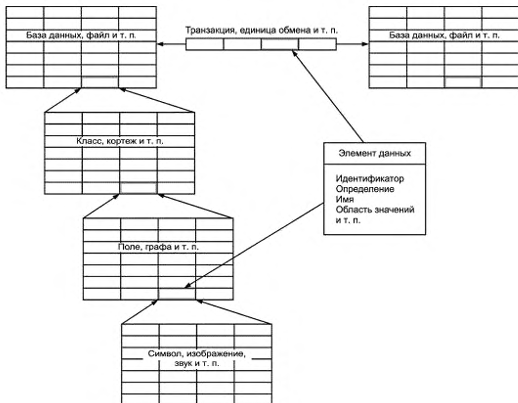
Рисунок 2 — Элементы данных и другие понятия
