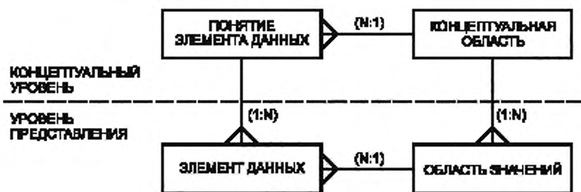
Рисунок 4 — Обзор модели РМД ИСО/МЭК 11179
