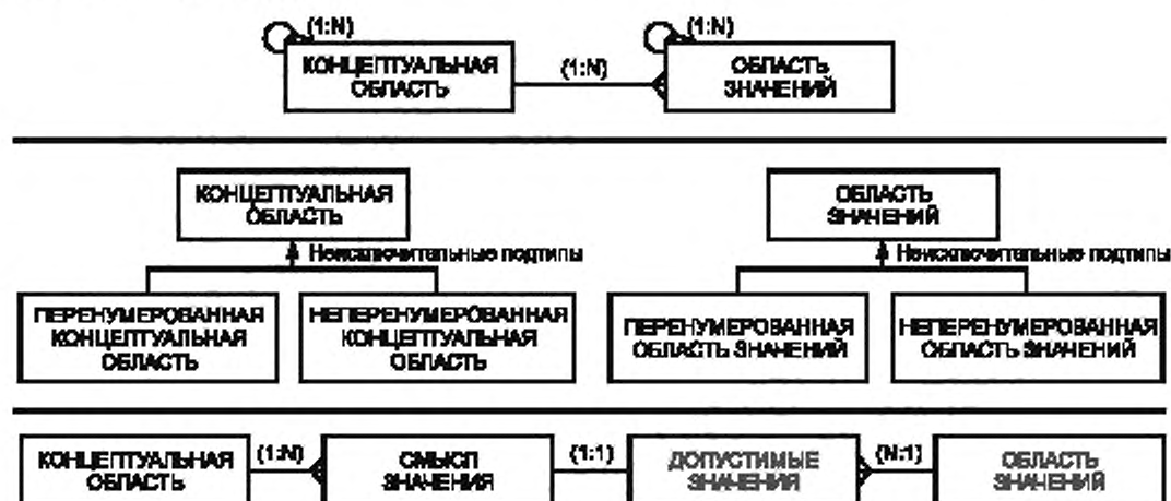
Рисунок 3 — Базовая модель областей значений
