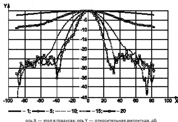
Рисунок А.2 — Характеристики направленности 0,2 мм — зондового гидрофона
