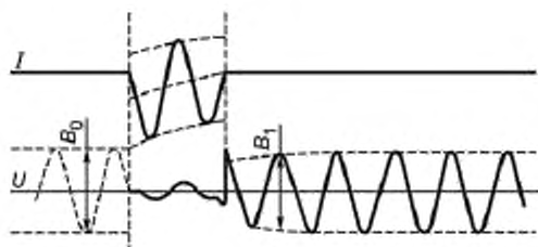
б) Осциллограмма отключения при образовании дуги после 180° с момента включения
