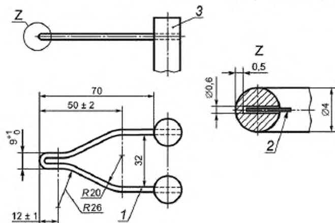
Рисунок 8 — Нагретая проволока и положение термопары
