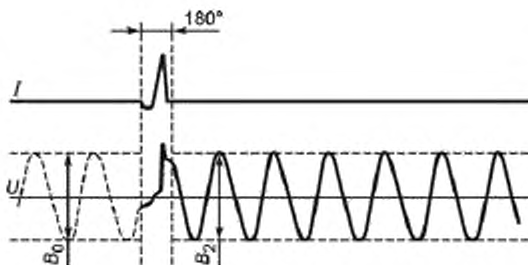
в) Осциллограмма отключения при образовании дуги до 180° с момента включения
