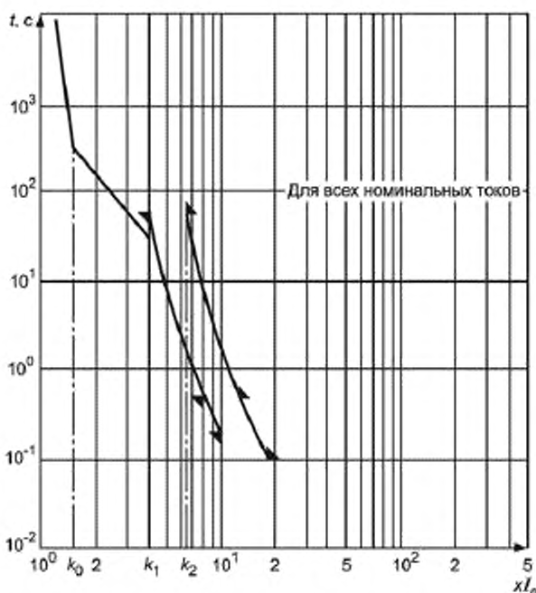
Рисунок 3 — Времятоковая зона плавких предохранителей «aM»
