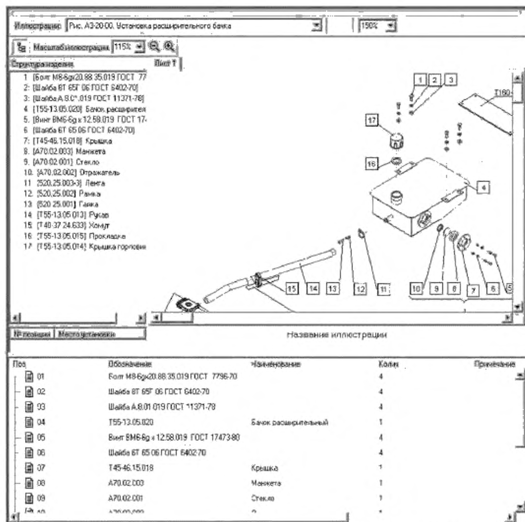
Рисунок Е.2 — Пример выполнения совмещенной формы, включающей отглавление, перечень деталей и иллюстрацию
