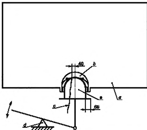
а — термокамера; б — образец для испытаний; с — термометр; d — подъемное устройство; e — термомакет головы
