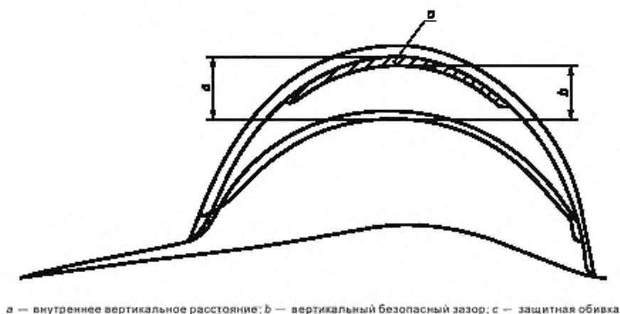
Рисунок 1 — Внутреннее вертикальное расстояние и вертикальный безопасный зазор
