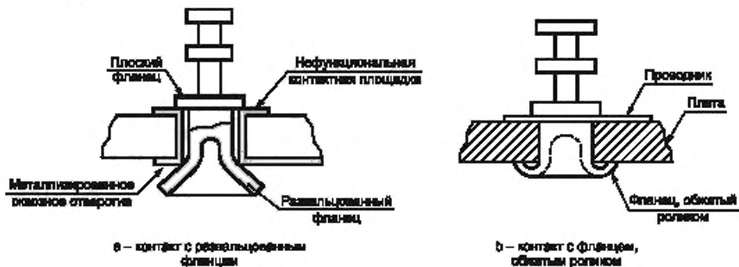
Рисунок 14 — Примеры закрепления контактов
