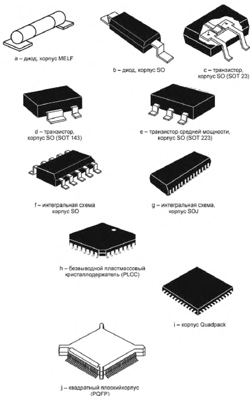
Рисунок 7 — Типовые конструкции корпусов полупроводниковых компонентов поверхностного монтажа
