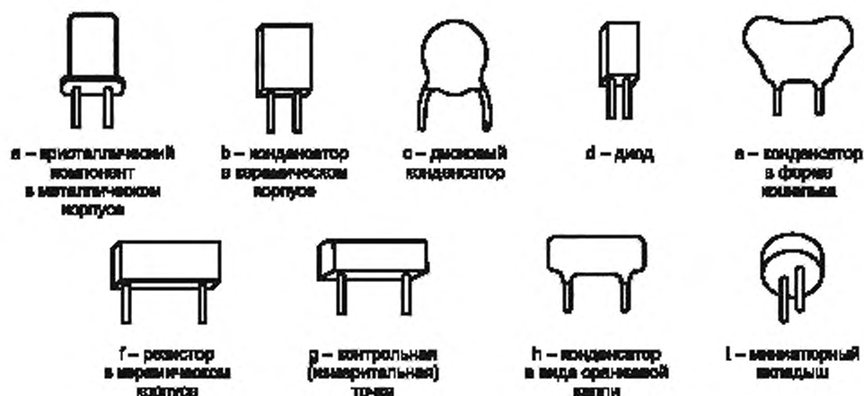
Рисунок 9 — Типовые компоненты с двумя радиальными выводами
