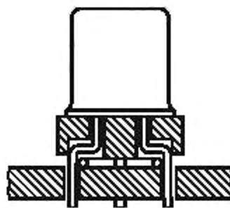
Рисунок 11 — Типовой транзистор с радиальными выводами на установочной панели
