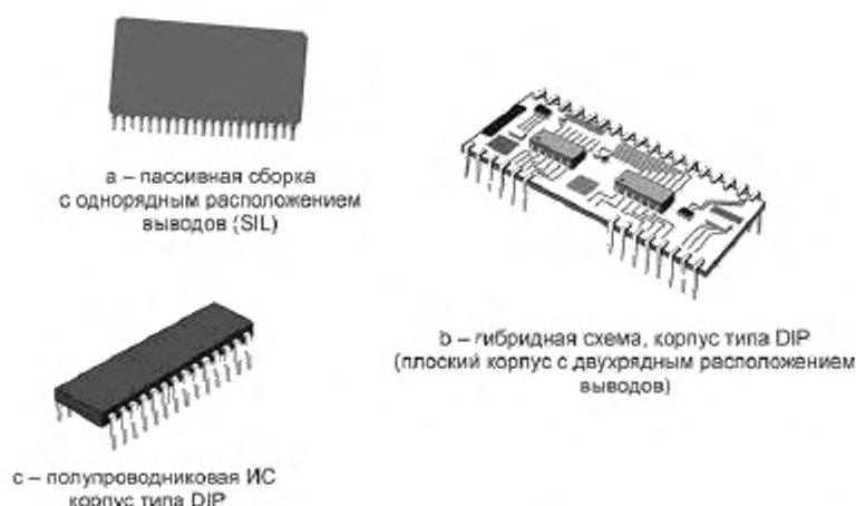
Рисунок 12 — Типовые конструктивные исполнения многовыводных корпусов ИС
