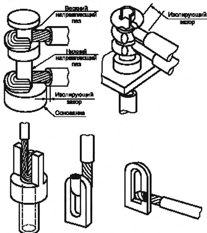
Рисунок 15 — Виды закрепления провода
