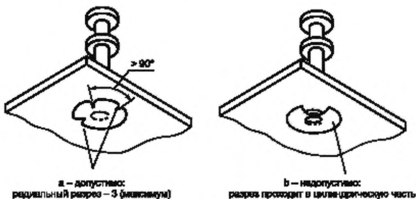
Рисунок 2 — Разрывы развальцованного фланца, обжатого руликом
