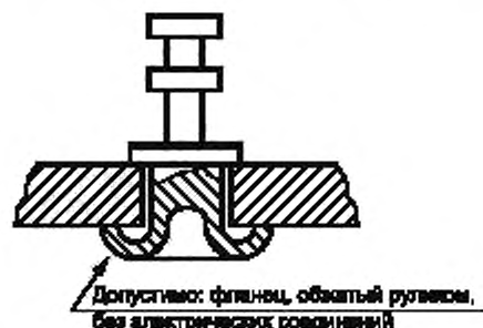
Рисунок 1 — Контакт с развальцованным фланцем
