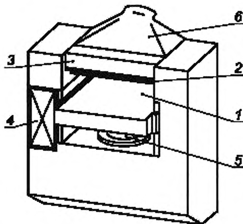
1 — загрузочный стол; 2 — устройство противоотдачи из качающихся планок; 3 — верхнее ограждение; 4 — панель управления; 5 — система подъема стола; 6 — вытяжной кожух
