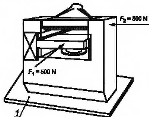
1 — древесностружечная плита
