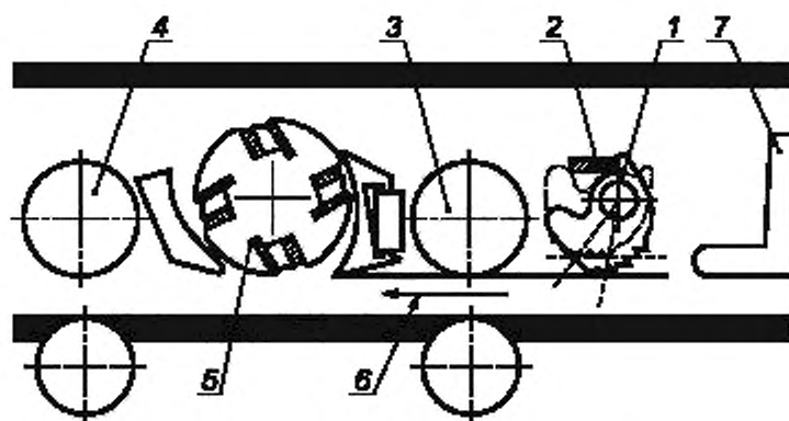
1 — устройство предотвращения качения планок; 2 — стопор для качающейся планки; 3 — приводной подающий ролик на входе; 4 — приводной подающий ролик на выходе; 5 — ножовой вал; 6 — направление подачи; 7 — устройство, ограничивающее толщину срезаемого слоя
